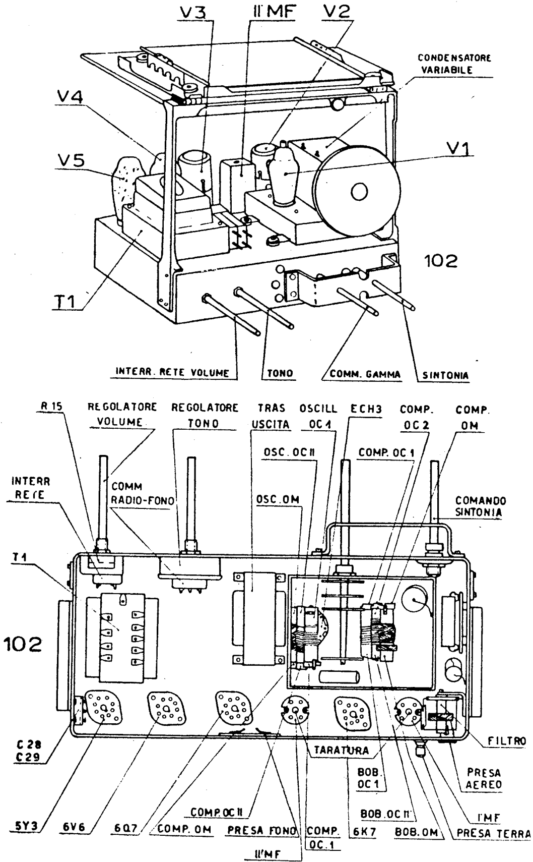
Prospetto e pianta del « 520 »
